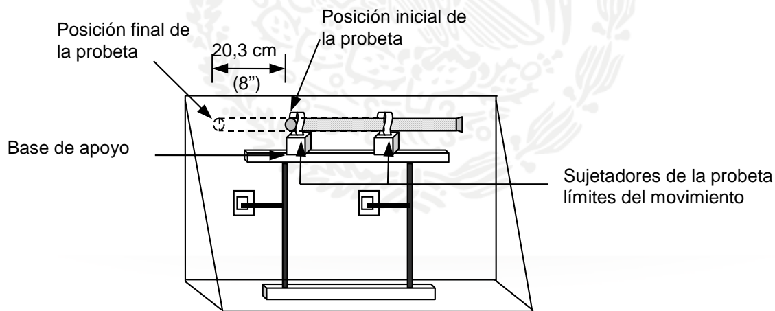
FIGURA 4.- Agitador manual
