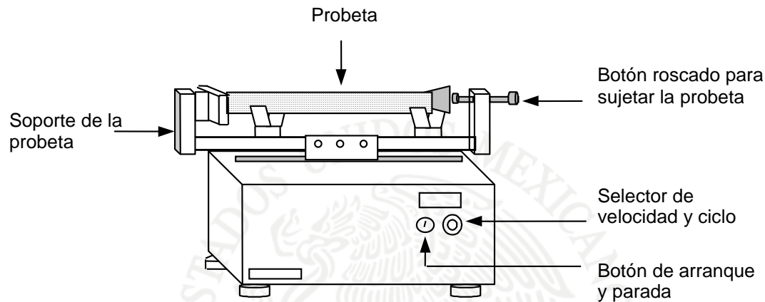
FIGURA 3.- Agitador mecánico
