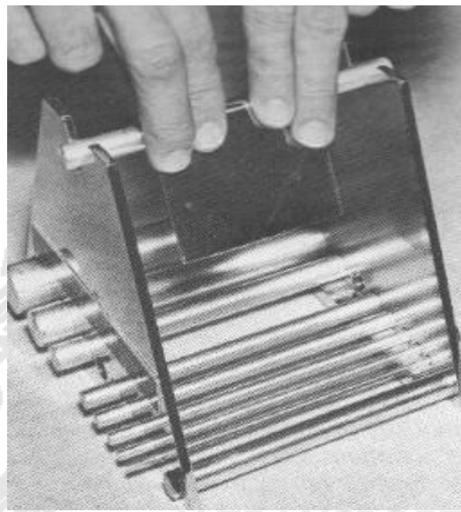
FIGURA 2.- Mandriles para la prueba de flexibilidad
