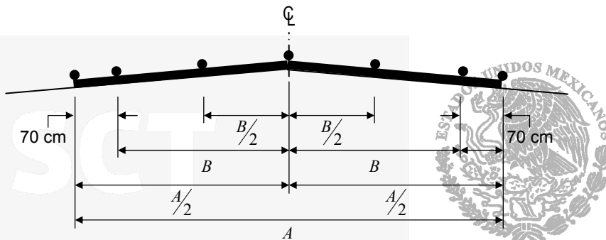
FIGURA 1.- Ubicación de los puntos por nivelar
