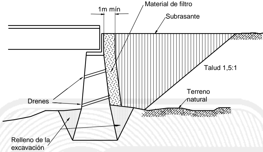
FIGURA 1.- Cuña de terraplén
