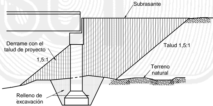
FIGURA 1.- Cuña de terraplén
