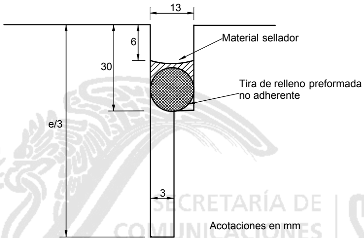
Detalle de la junta
