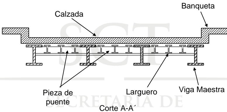
FIGURA 1.- Detalle de pieza de puente
