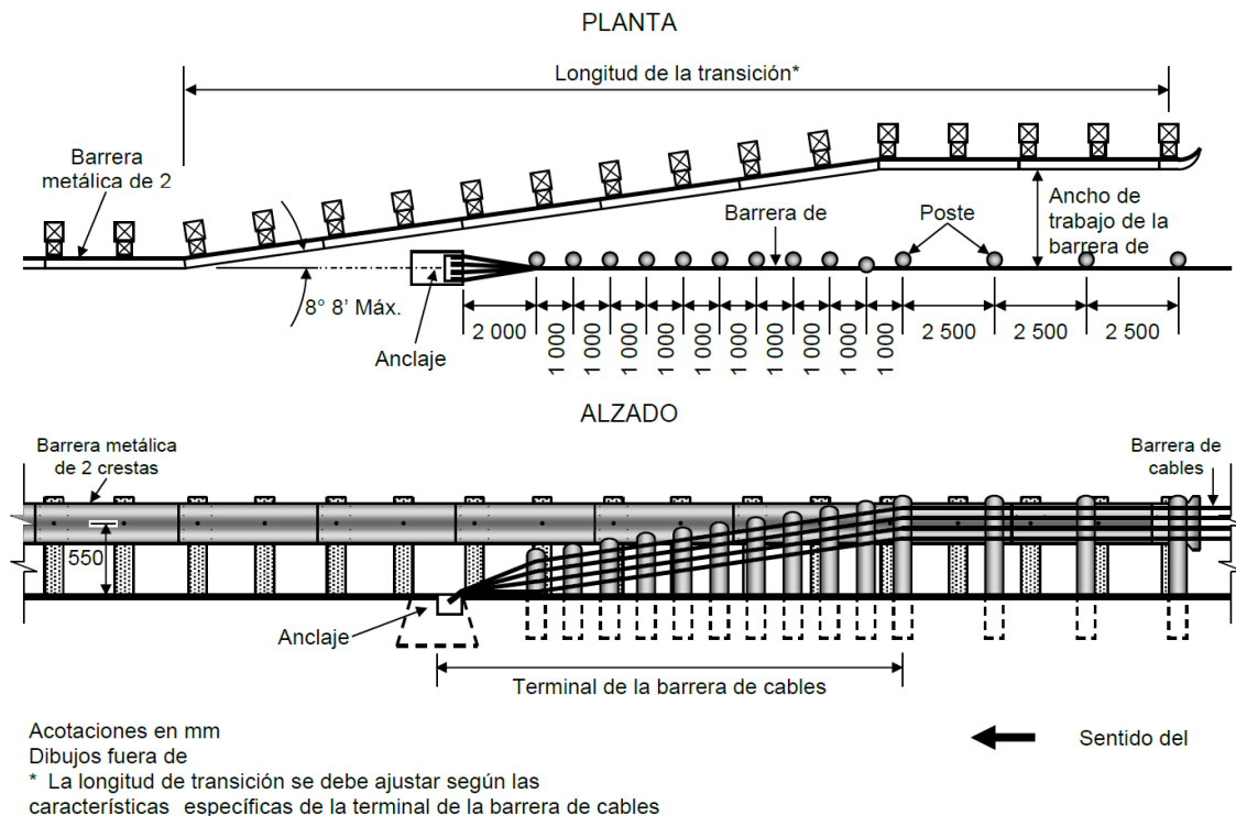
FIGURA 25.- Transición de barrera flexible de cables de acero
