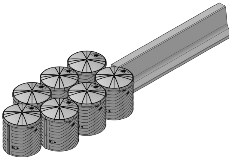
FIGURA 27.- Sección de amortiguamiento no redireccionable (OD-4.4.1/NR)
