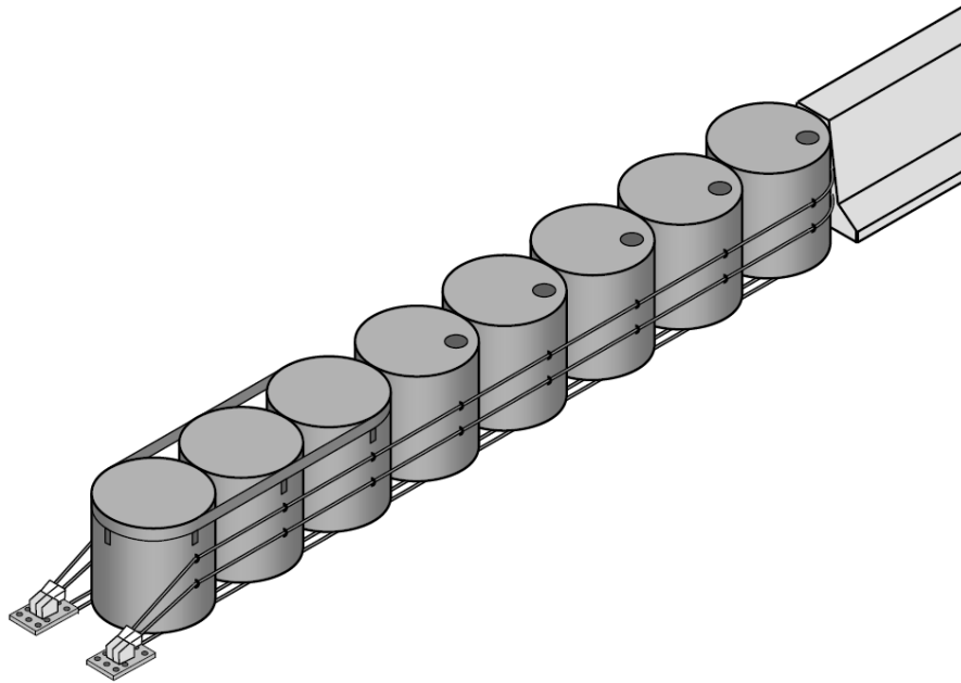
FIGURA 26.- Sección de amortiguamiento redireccionable-traspasable (OD-4.4.1/RT)
