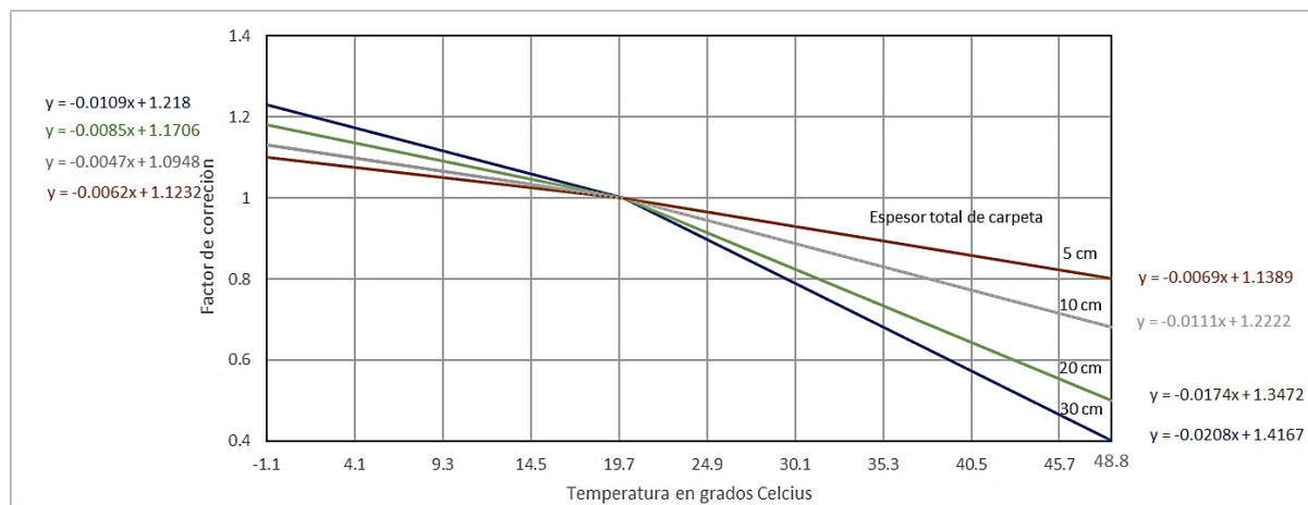
FIGURA 3.- Gráfico para determinación del factor de corrección de deflexiones por temperatura para pavimentos con bases estabilizadas con cemento
