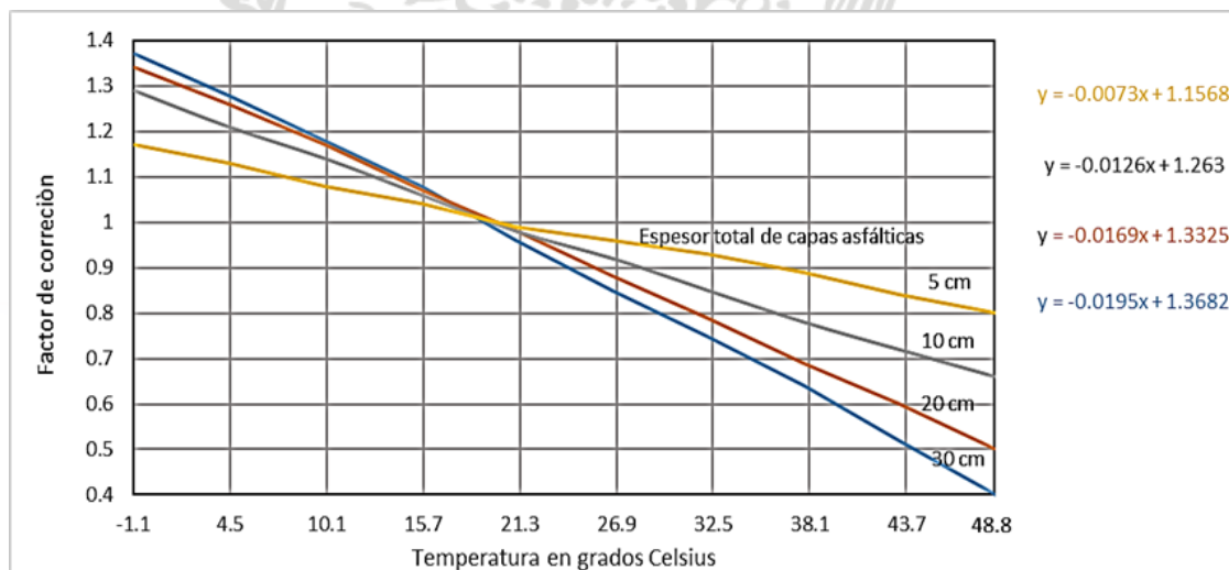
FIGURA 2.- Gráfico para determinación del factor de corrección de deflexiones por temperatura para pavimentos con bases hidráulicas o estabilizadas con asfalto y/o cal
