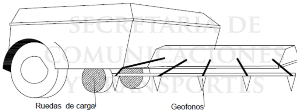
FIGURA 1.- Equipo de medición dinámica remolcado por un vehículo
