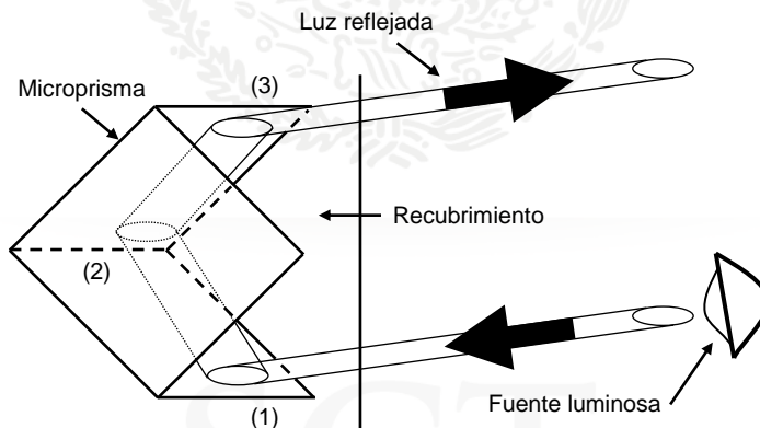
FIGURA 2.- Fenómeno de reflexión en una película reflectante con microprismas
