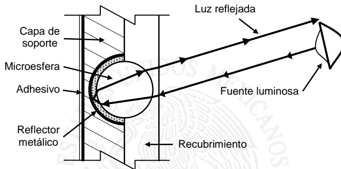
FIGURA 1.- Fenómeno de reflexión en una película reflectante con microesferas
