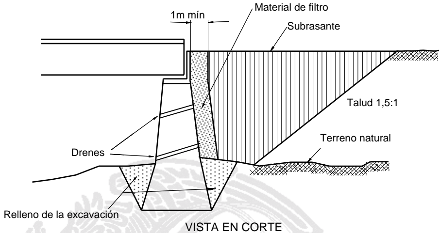
FIGURA 1.- Cuña de terraplén
