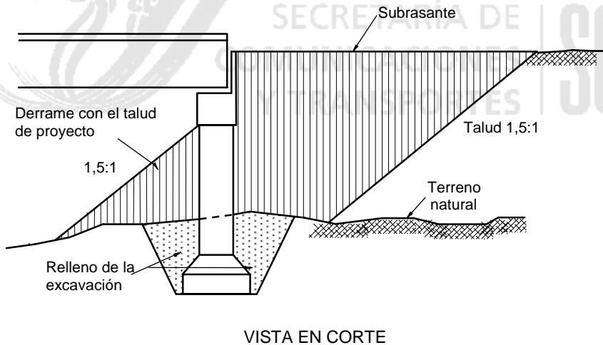
FIGURA 2.- Cuña de terraplén con derrame
