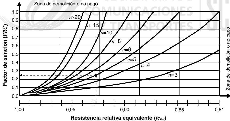
FIGURA 1.- Gráfica para determinar el factor de sanción por resistencia insuficiente del concreto lanzado ( FRC )
