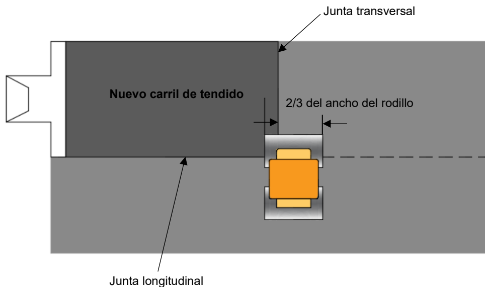
FIGURA 1.- Traslape con compactador de rodillo
