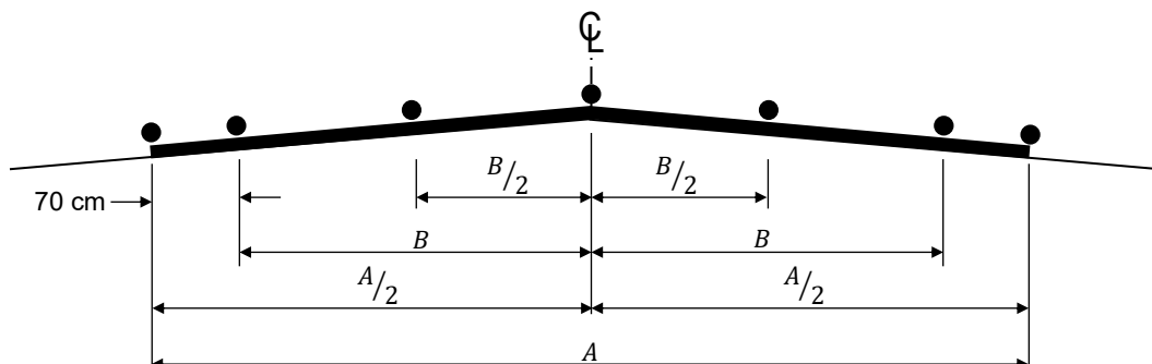
FIGURA 2.- Ubicación de los puntos por nivelar
