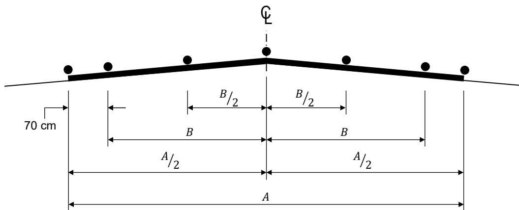
FIGURA 2.- Ubicación de los puntos por nivelar
