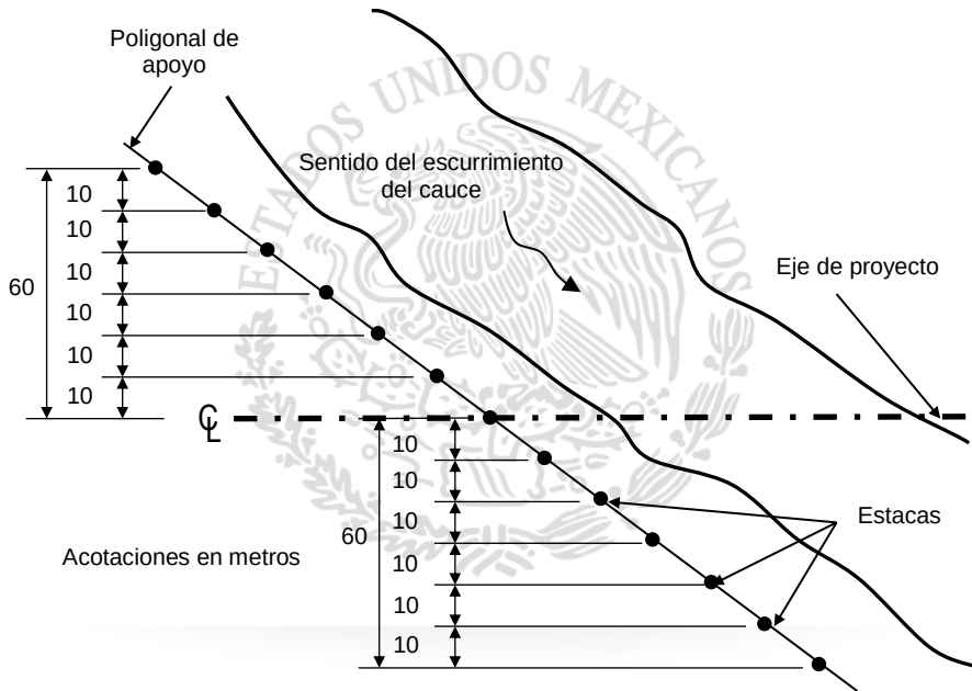
FIGURA 1.- Ubicación de las estacas sobre la poligonal de apoyo para sustentar las secciones topográficas para la Planta Detallada
